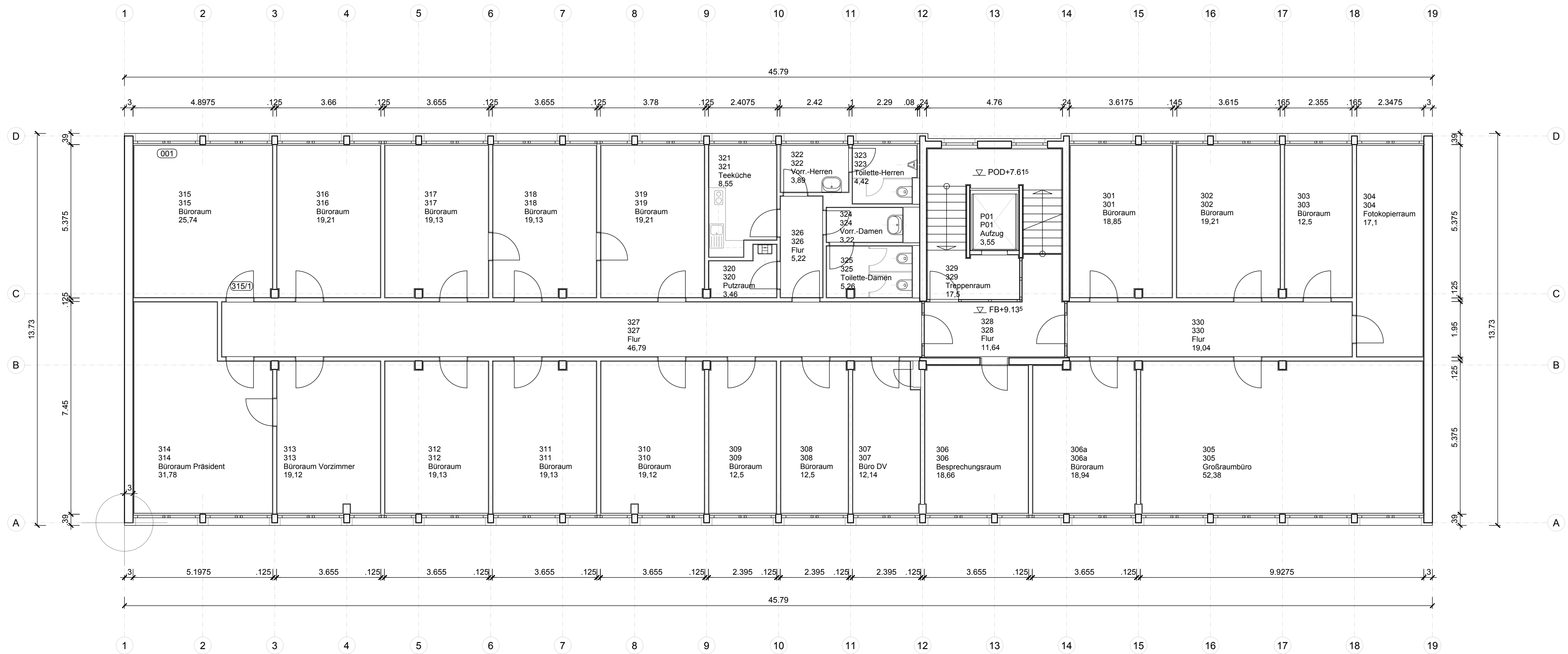
GRUNDRISS 3. OBERGESCHOSS
